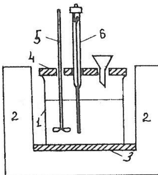
Рисунок 3.1 – Изотермический калориметр
