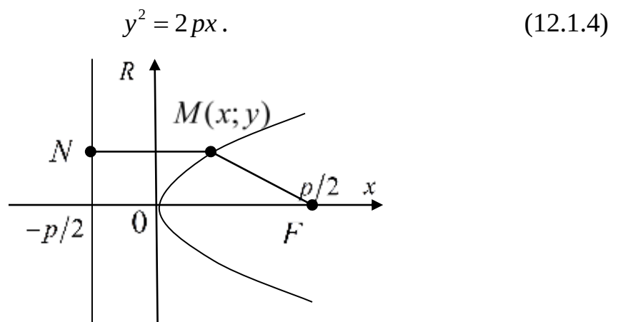
Рисунок 12.1.4 – Парабола
