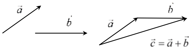
Рисунок 3.1.3 – Правило треугольника
