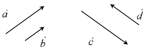
Рисунок 3.1.2 – Сонаправленность
