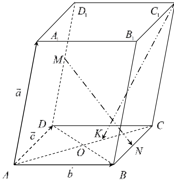
Рисунок 3.2.3 – Параллелепипед
