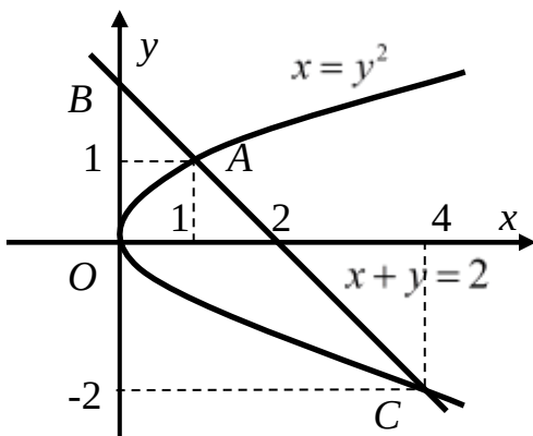
Рисунок 1.1 – Фигура OAC
