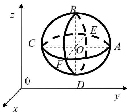
Рисунок 5.2 – Сфера
