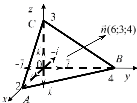
Рисунок 6.1 – Поток
