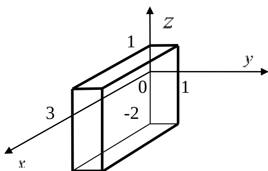
Рисунок 2.1 – Параллелепипед
