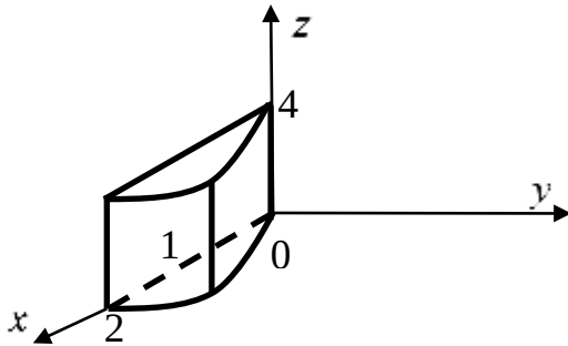
Рисунок 2.2 – Полуцилиндр
