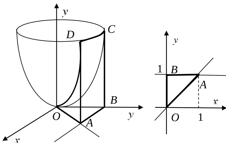
Рисунок 3.2 – Тело T_1 и его проекция на плоскость
