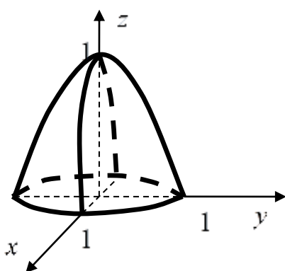
Рисунок 5.1 – Параболоид
